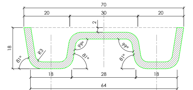
CORR. 'W' PALE SECTION DET.
